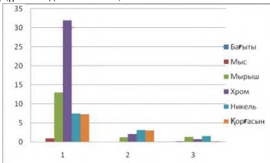
Сурет 1 - АФЗ аймағындағы топырақтардың ауыр металдармен ластануы
